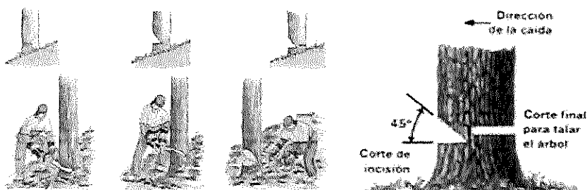
Figura 4. Guía para el descope de los árboles. Fuente: Tacha y Moreno, 2016.
