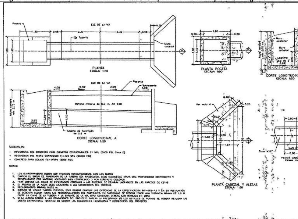
Figura 20. Planta Secciones Alcantarilla 36" Fuente: Municipio de la Jagua de Ibirico
