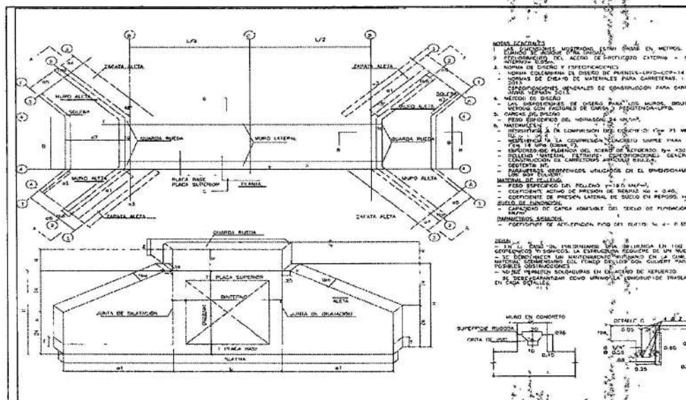
Figura 19. Geometría Box Culvert – Planta Frontal Fuente: Municipio de la Jagua de Ibirico
