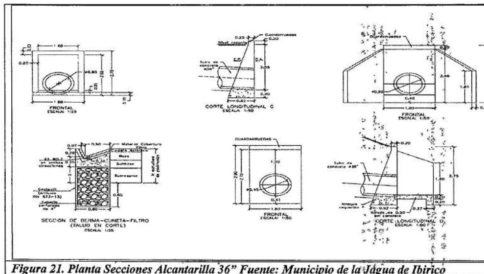
Figura 21. Planta Secciones Alcantarilla 36" Fuente: Municipio de la Jagua de Ibirico
