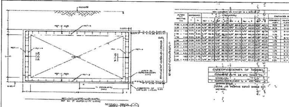
Figura 16. Planta Secciones Box Culvert Doble de 1.00 X 2.00 Fuente: Municipio de la Jagua de Ibirico
