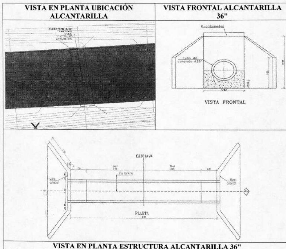
Imagen No. 4: Diseño alcantarilla de 36"
