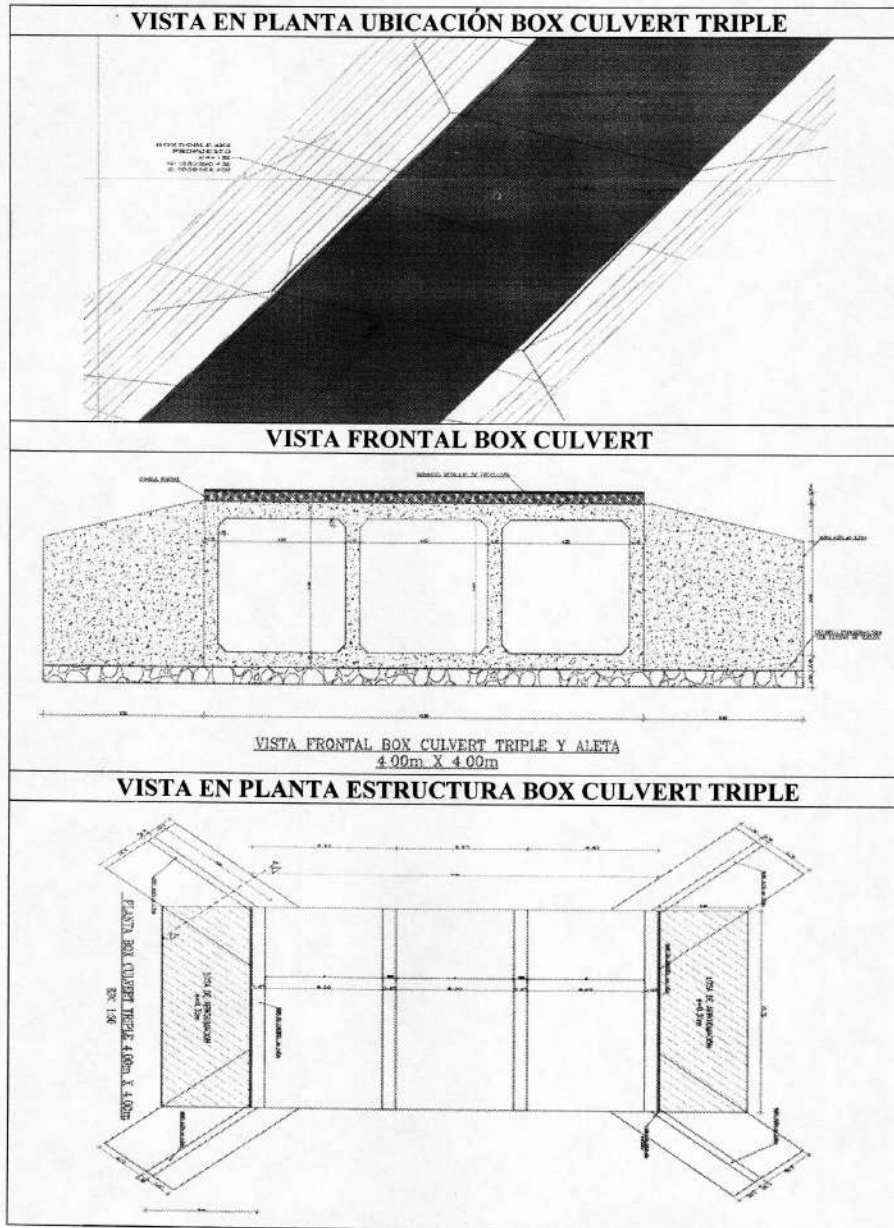
Imagen No. 6: Diseño Box Coulvert Triple
