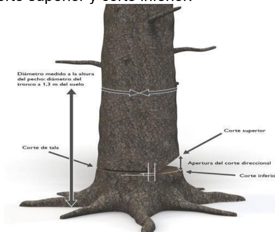
Ilustración 2. Corte de Tala
