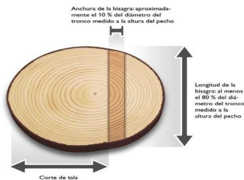
Ilustración 3. Apeo
