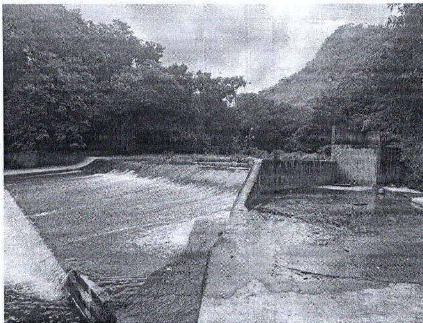
Imagen 4. Bocatoma sistema de acueducto de Becerril sobre el Río Socomba – Fuente: Propia.
