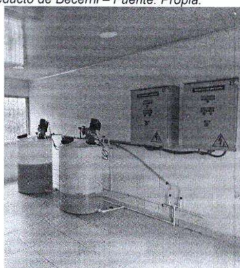
Imágenes 8 y 9. PTAP 1 y dosificación de Coagulante sistema de acueducto de Becerril – Fuente: Propia.
