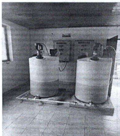
Imágenes 10 y 11. PTAP 2 y dosificación de coagulante sistema de acueducto de Becerril – Fuente: Propia.
