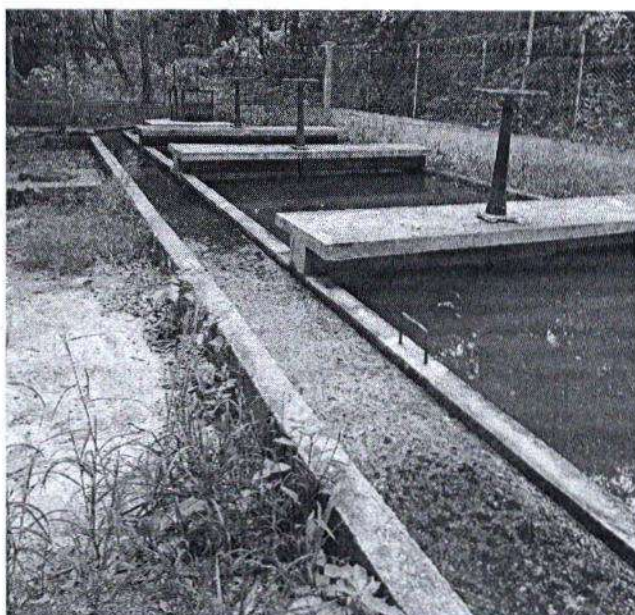
Imágenes 6 y 7. Desarenadores 1 y 2 sistema de acueducto de Becerril – Fuente: Propia.
