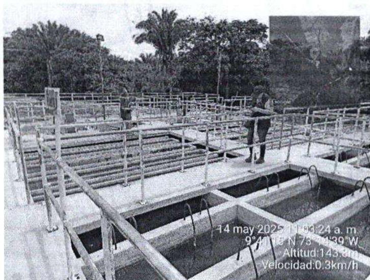
Imágenes 10 y 11. PTAP 2 y dosificación de coagulante sistema de acueducto de Becerril – Fuente: Propia.
