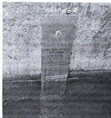
Imágenes 14 y 15. Regletas para la lectura de la altura de la lámina de agua y la determinación del caudal – Fuente: Propia.
