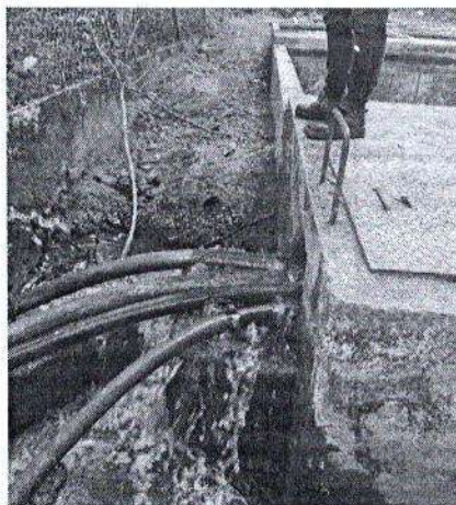
Imagen 13. Conexiones no autorizadas en el desarenador a través de mangueras para predios particulares – Fuente: Propia.
