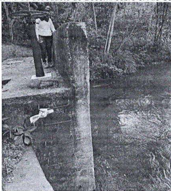
Imagen 5. Bocatoma sistema de acueducto de Becerril sobre el Río Maracas – Fuente: Propia.
