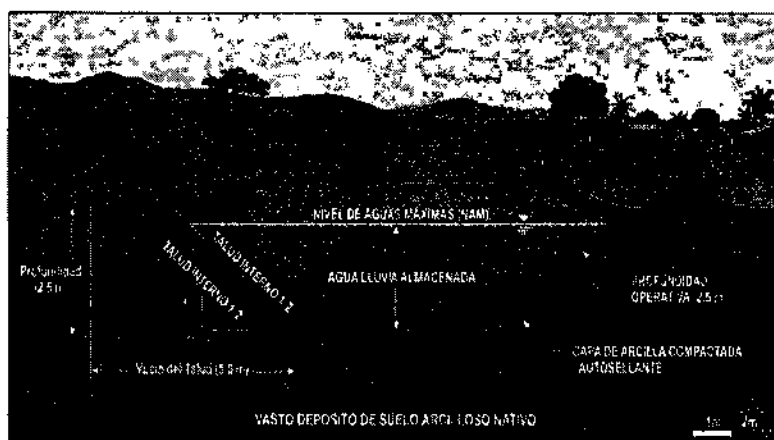
Figura 4 Diseño general de Jagüey
