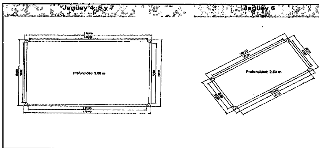
Figura 2. Dimensiones jagüeyes 4, 5, 6 y 7
