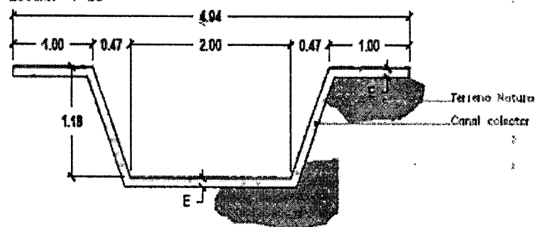
Imagen 8. Colector pluvial E sobre el río San Alberto
