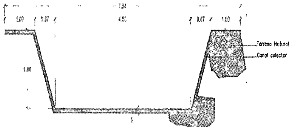
SECCIÓN TRANSVERSAL TIPO CANAL COLECTOR TRAMO III. Escala: 1: 50
