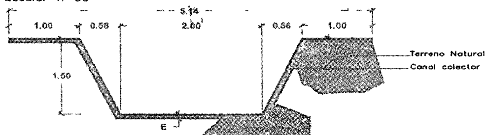
Imagen 6. Canal pluvial 2 a Box
