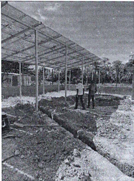
Paneles solares y centro de control
